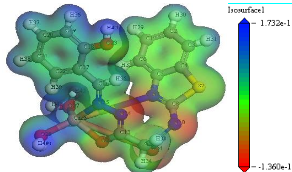
[Cu(BT)(H 2 O) 2 ].2H 2 O
